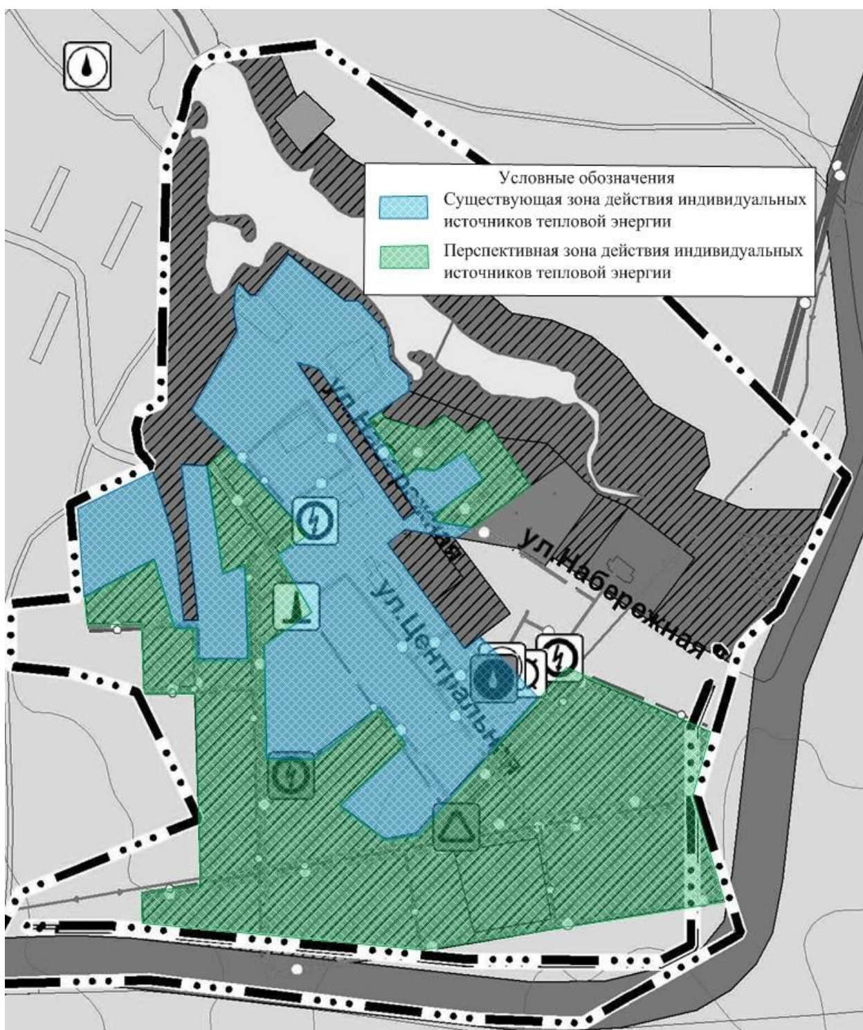
Рис. № 27 - Существующие и перспективные зоны действия индивидуального теплоснабжения на территории п. Кочевой
