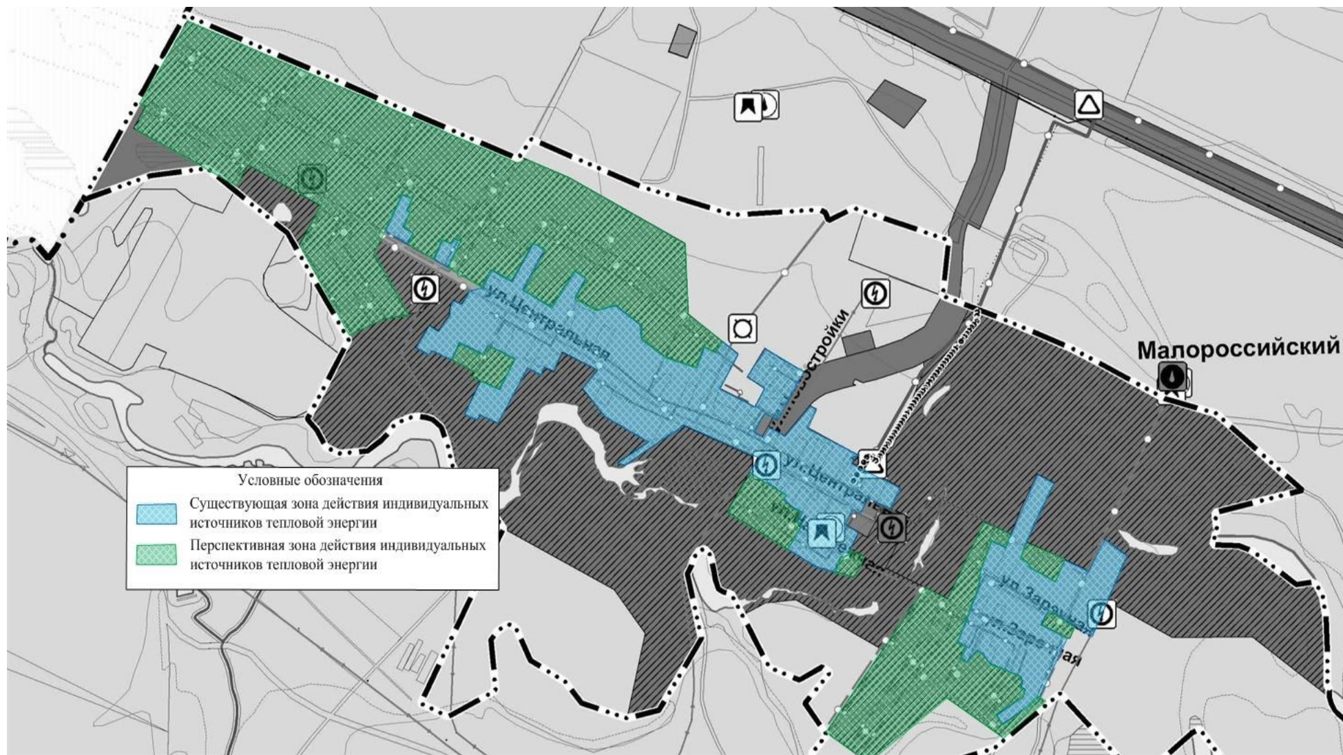
Рис. № 22 - Существующие и перспективные зоны действия индивидуального теплоснабжения на территории п. Малоросийский
