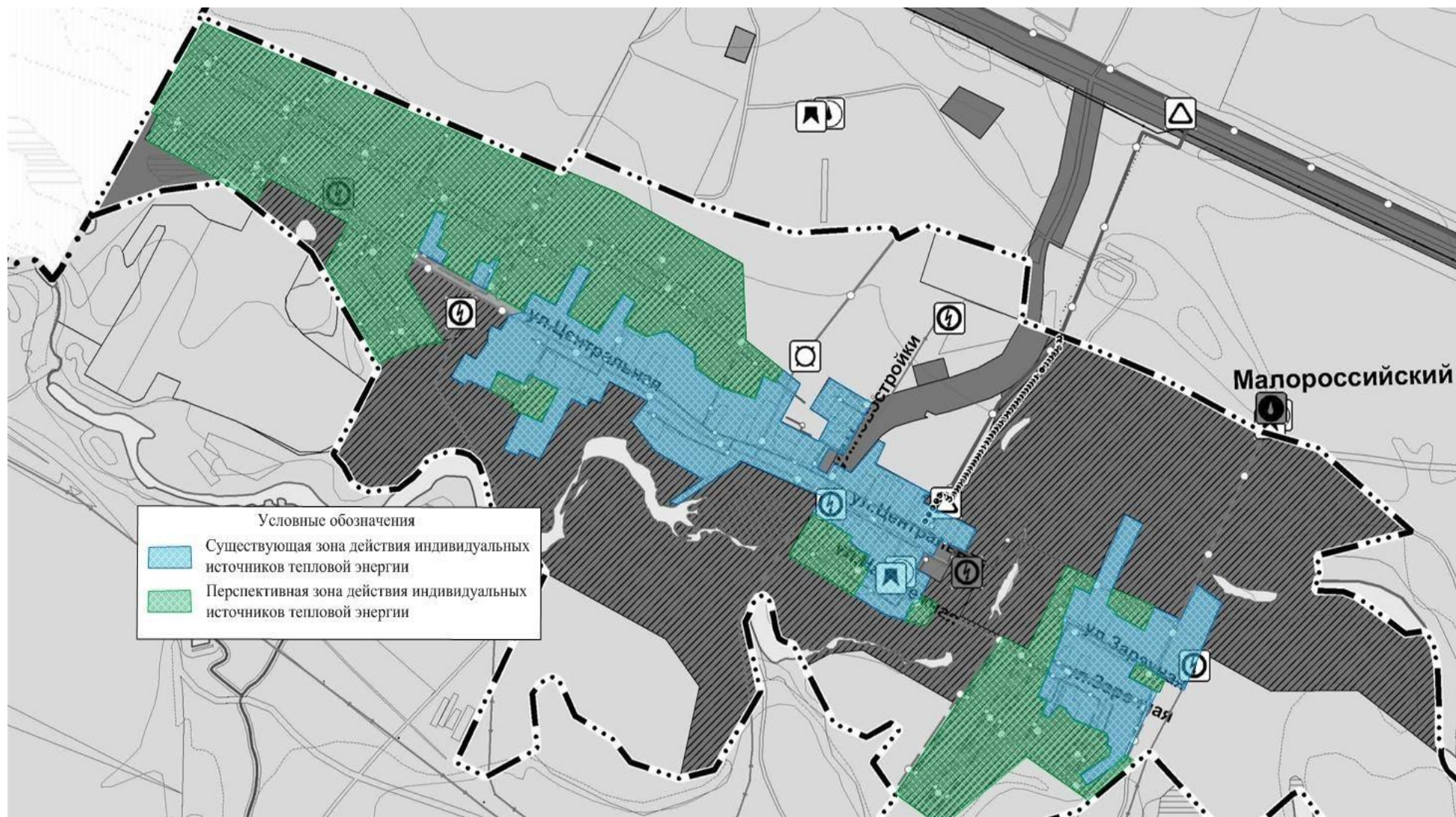
Рис. № 22 - Существующие и перспективные зоны действия индивидуального теплоснабжения на территории п. Малороссийский
